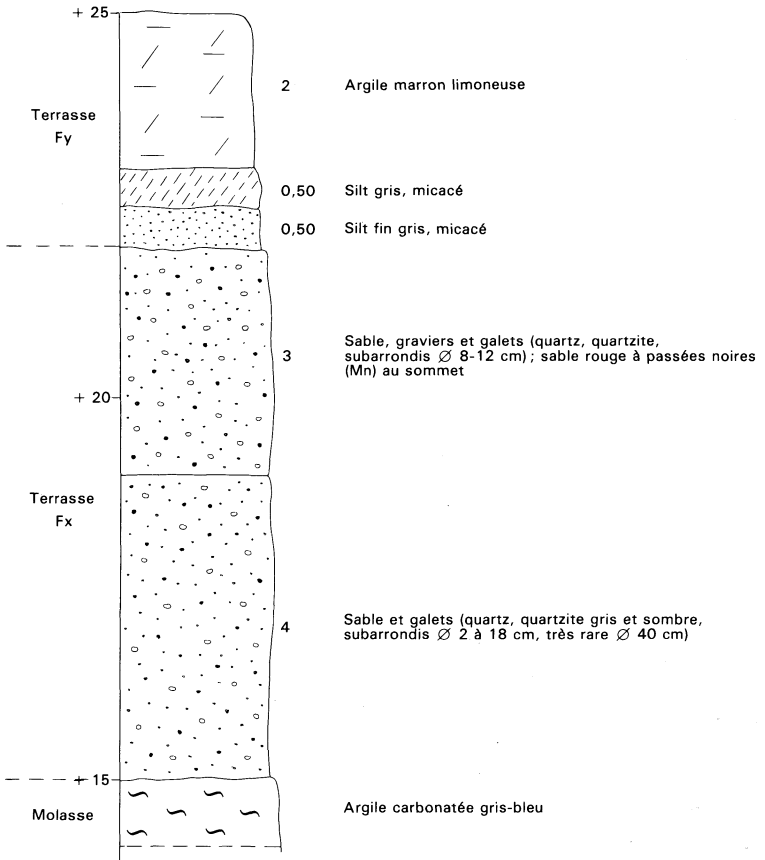
Fig. 9 - Coupe de Borde-Vieille (front de la carrière du lieu-dit Borde-Vieille et forage 877-8-10, commune de Lagruère)
