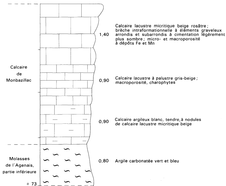
Fig. 2 - Coupe du lac de Clarens (D. 933, lieu-dit Maynéou, commune de Casteljalous)
