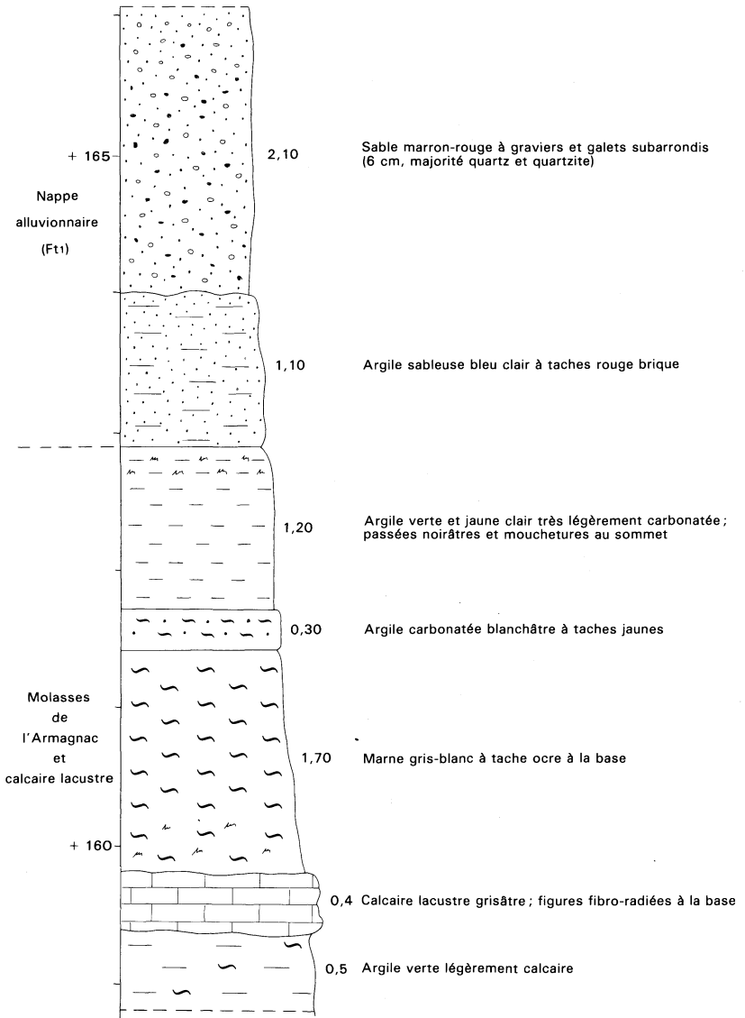
Fig. 5 - Coupe du château d'eau de Labastide-Castelamoureux (D. 6, commune de Labastide-Catelamoureux)
