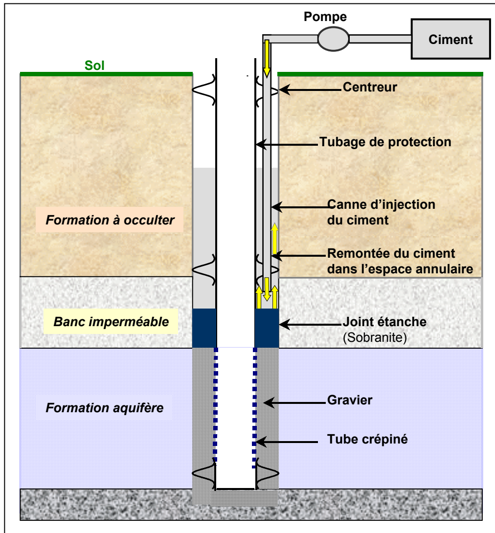
Illustration 12 - Cimentation par canne (schéma n°2) Source documentaire BRGM
