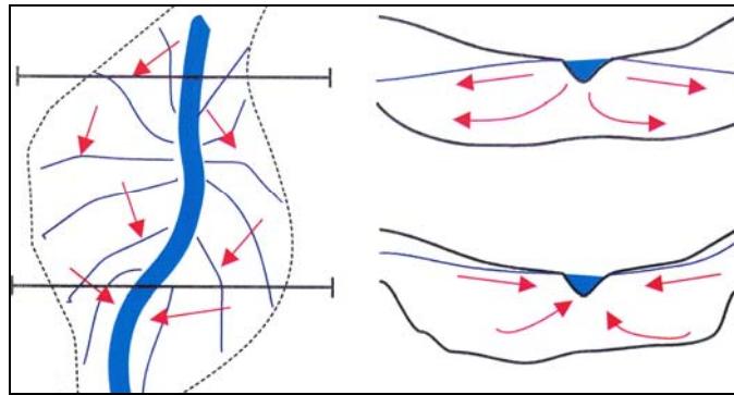
Illustration 33 - Exemple de relations nappe - rivière
