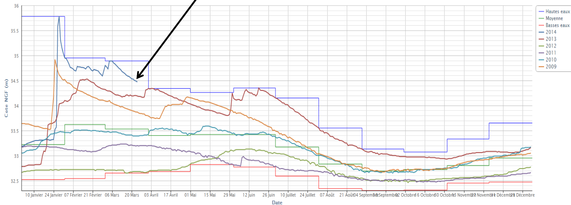
Graphique du piézomètre 09021X0120/PZ – LA CROIX DE SABAROS (SAINT-LAURENT - 47)
