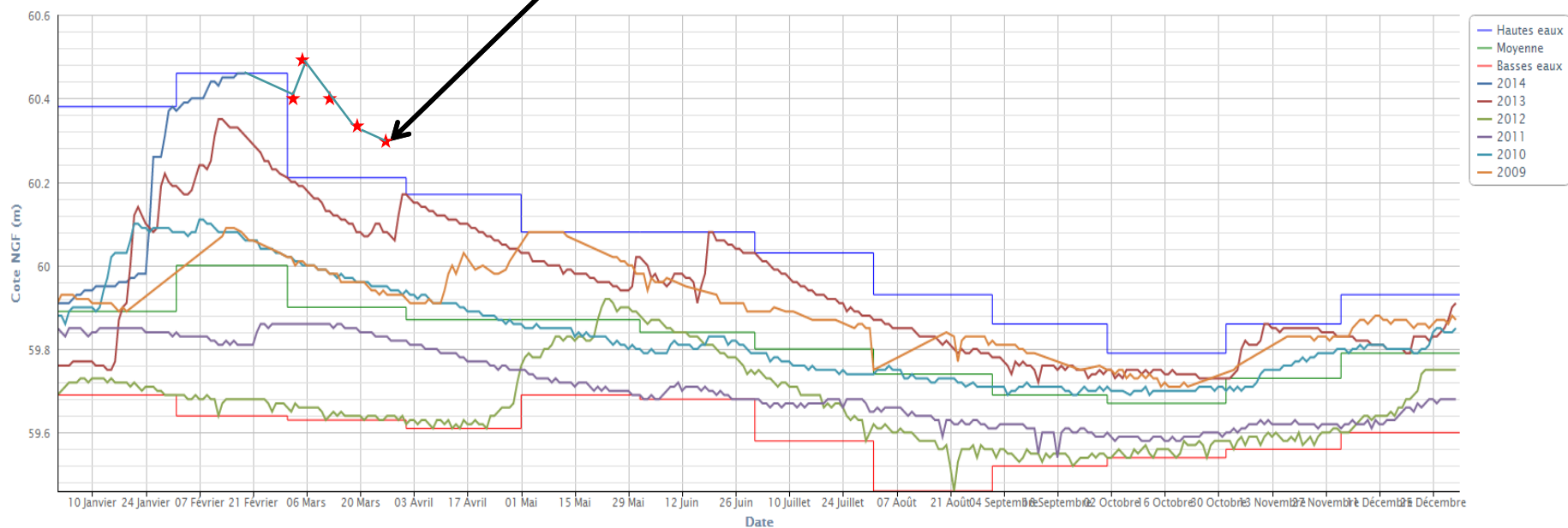
Graphique du piézomètre 08791X0031/P3 – LA BOURDETE (VILLENEUVE-SUR-LOT - 47)
