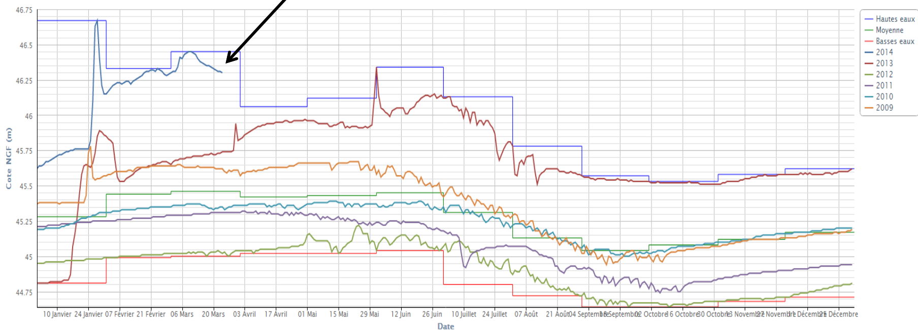
Graphique du piézomètre 09028X0071/P – LE PONT (SAUVETERRE-SAINT-DENIS - 47)
