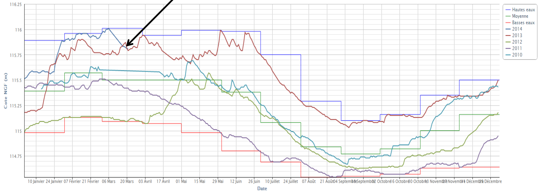
Graphique du piézomètre 09012X0027/PZ – CAMPET (DURANCE - 47)
