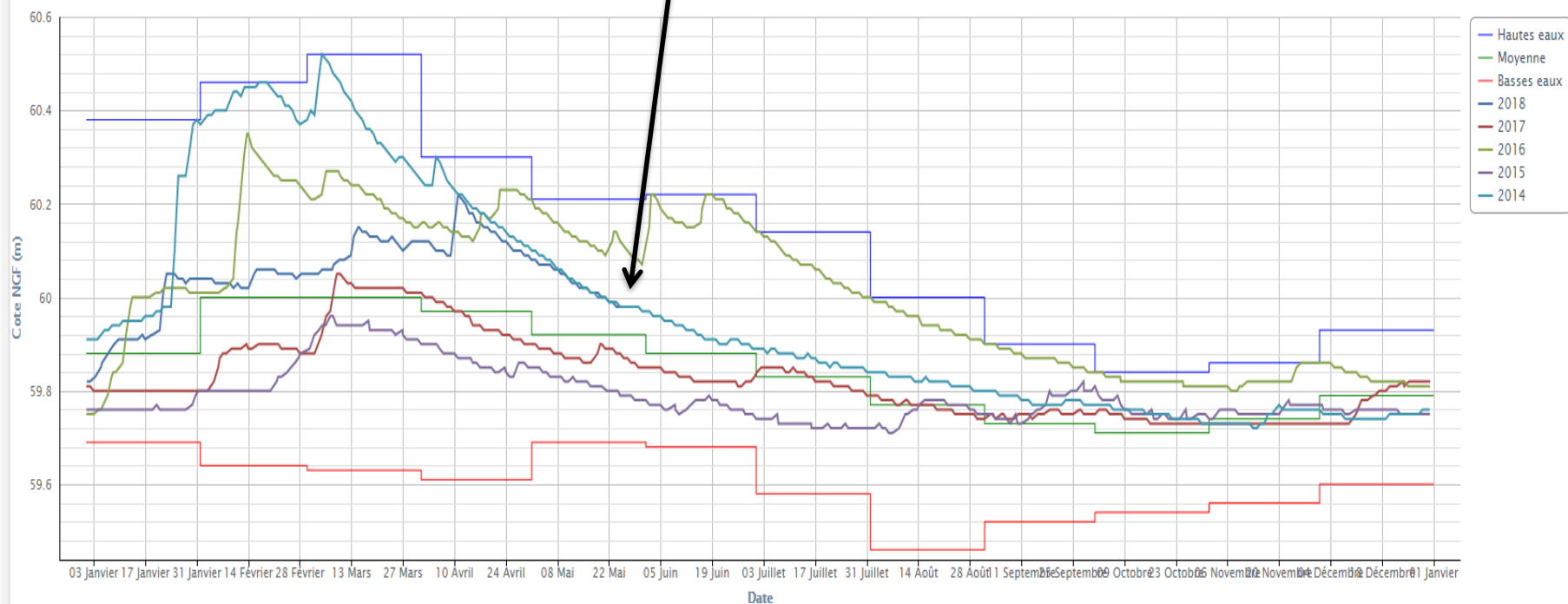
Graphique du piézomètre 08791X0031/P3 – LA BOURDETE (VILLENEUVE-SUR-LOT - 47)
