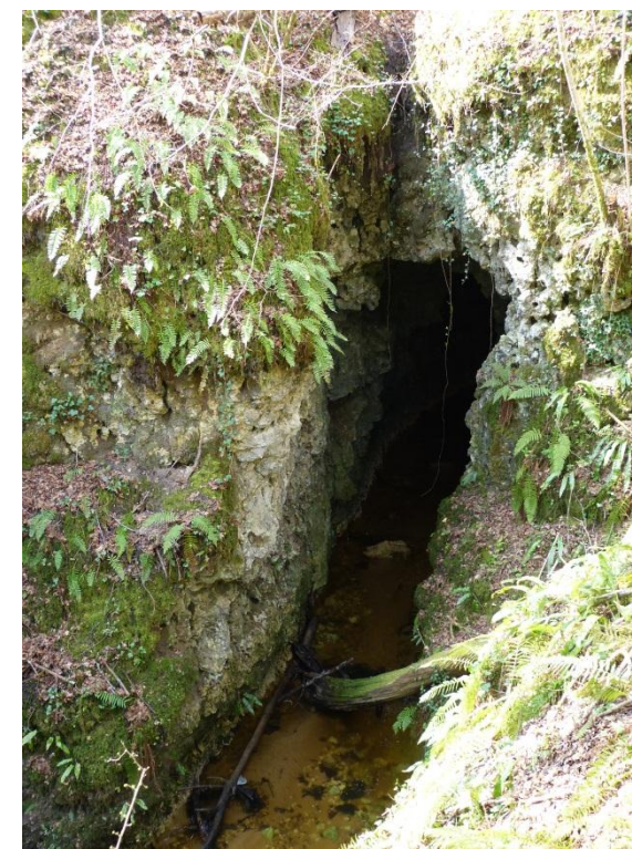
Figure 3 : Entrée d'une galerie karstique sur faille ouverte, d'où s'écoule le ruisseau du Cros (Platel JP., 2014)
